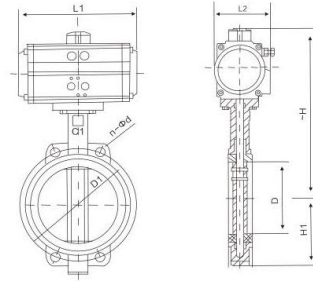
尺寸size(mm)
